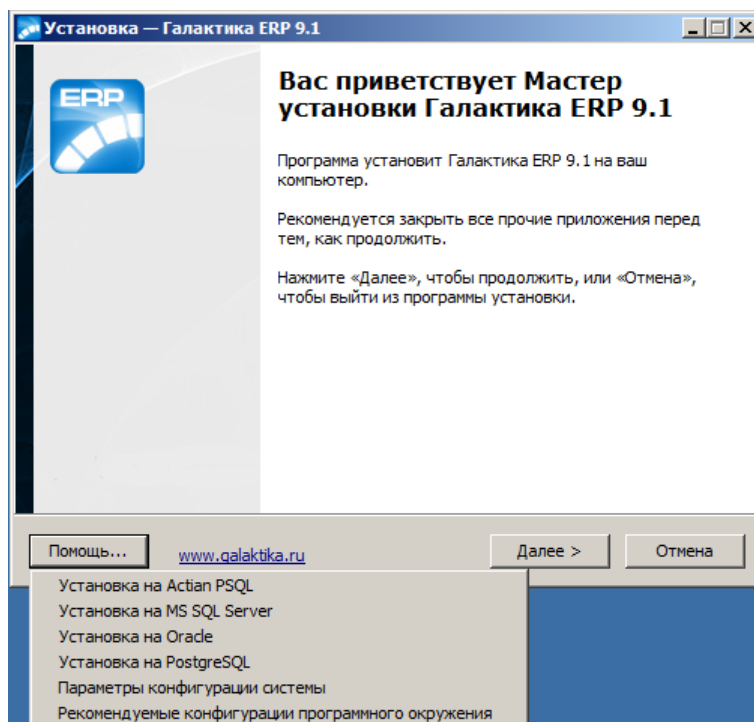
Рис. 13. Окно приветствия
