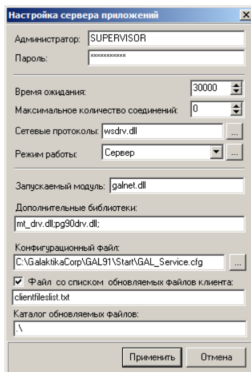
Рис. 42. Окно «Настройка сервера приложений»
